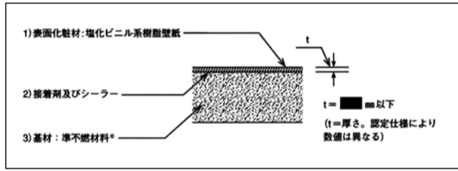
石こうボード・石膏ボード面の下地調整標準施工図
