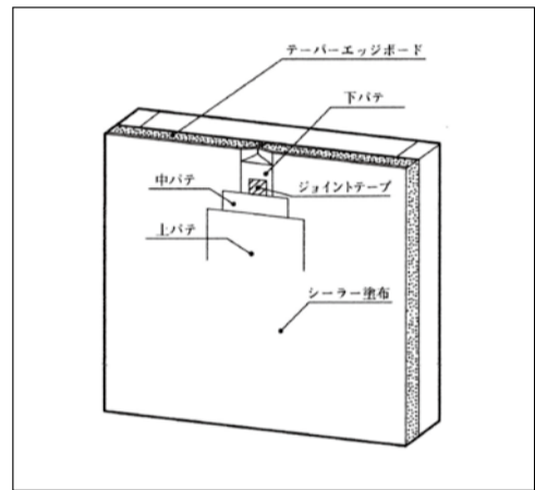
せっこうボードテーパード面の下地調整標準施工図
