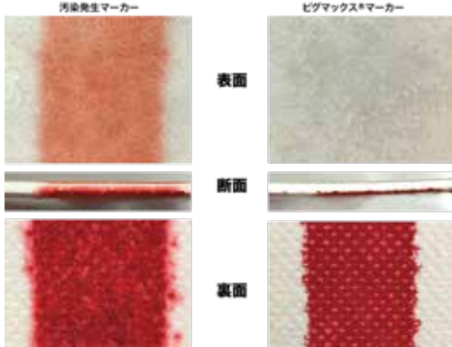
床材汚染場面図 床材の裏面にマーキングし、40℃1週間加熱(促進試験)
