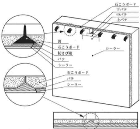
石こうボード・ベベルボード面の下地調整標準施工図
